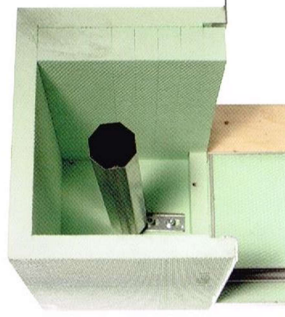
Sezione del cassonetto termoisolante Isolbox nella versione "ultra", con doppio pannello isolante all'interno.
