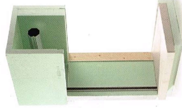
Dettaglio della sezione della spalla laterale. Si nota che la guida ed il profilo di giunzione del falso telaio sono sporgenti di 3 mm per lasciar spazio alla rasatura e alla decorazione finale in tono con le pareti.
